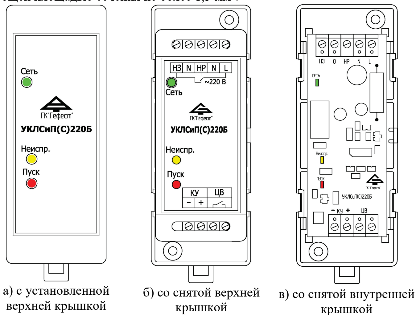
Рисунок 1. Внешний вид УКЛСиП(С)220Б
